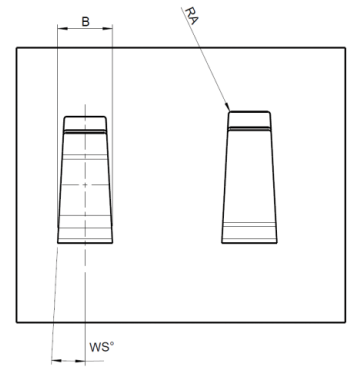
without clearance / ohne Freistanzung
