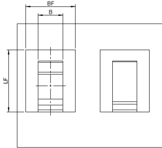
with clearance / mit Freistanzung
